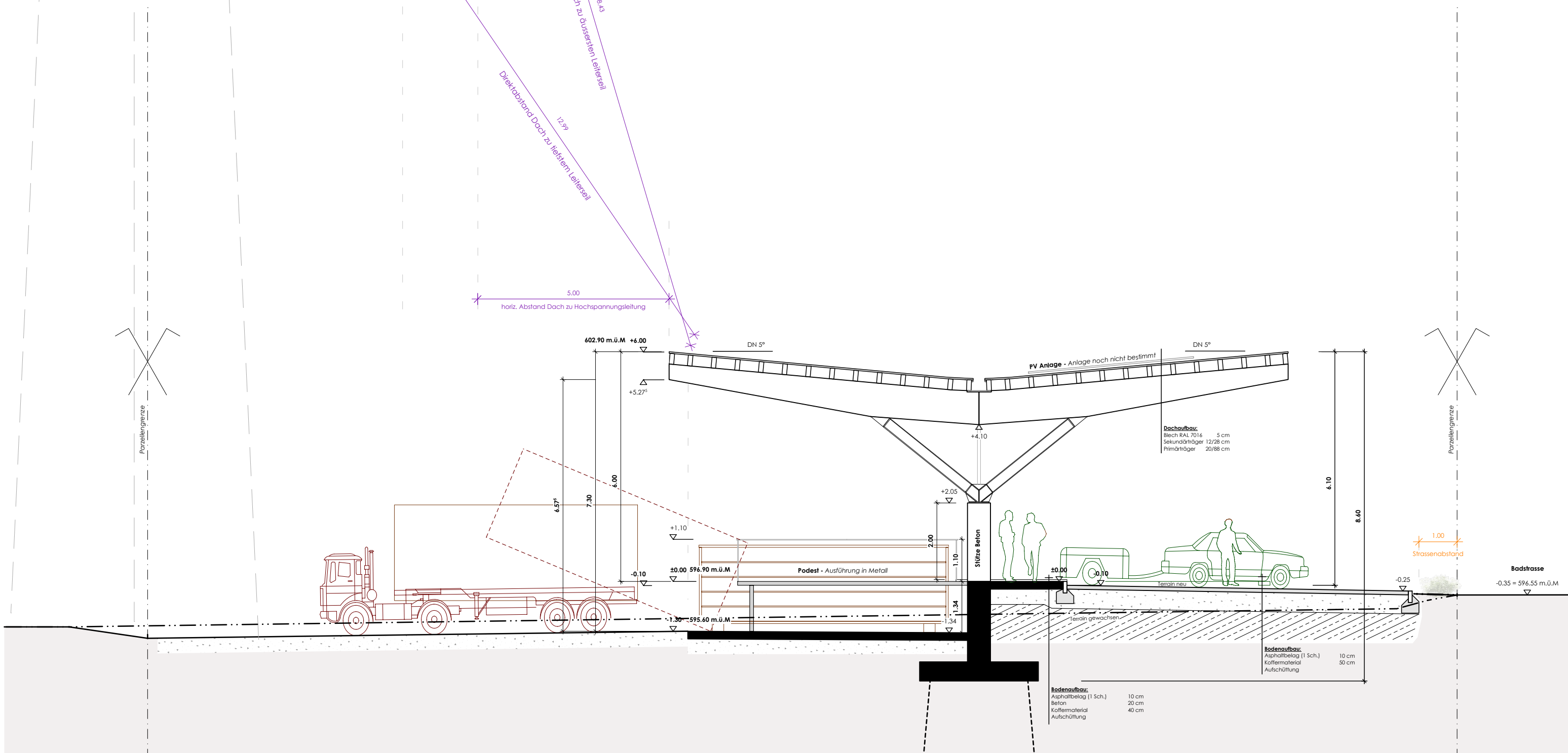
Querschnitt 1
