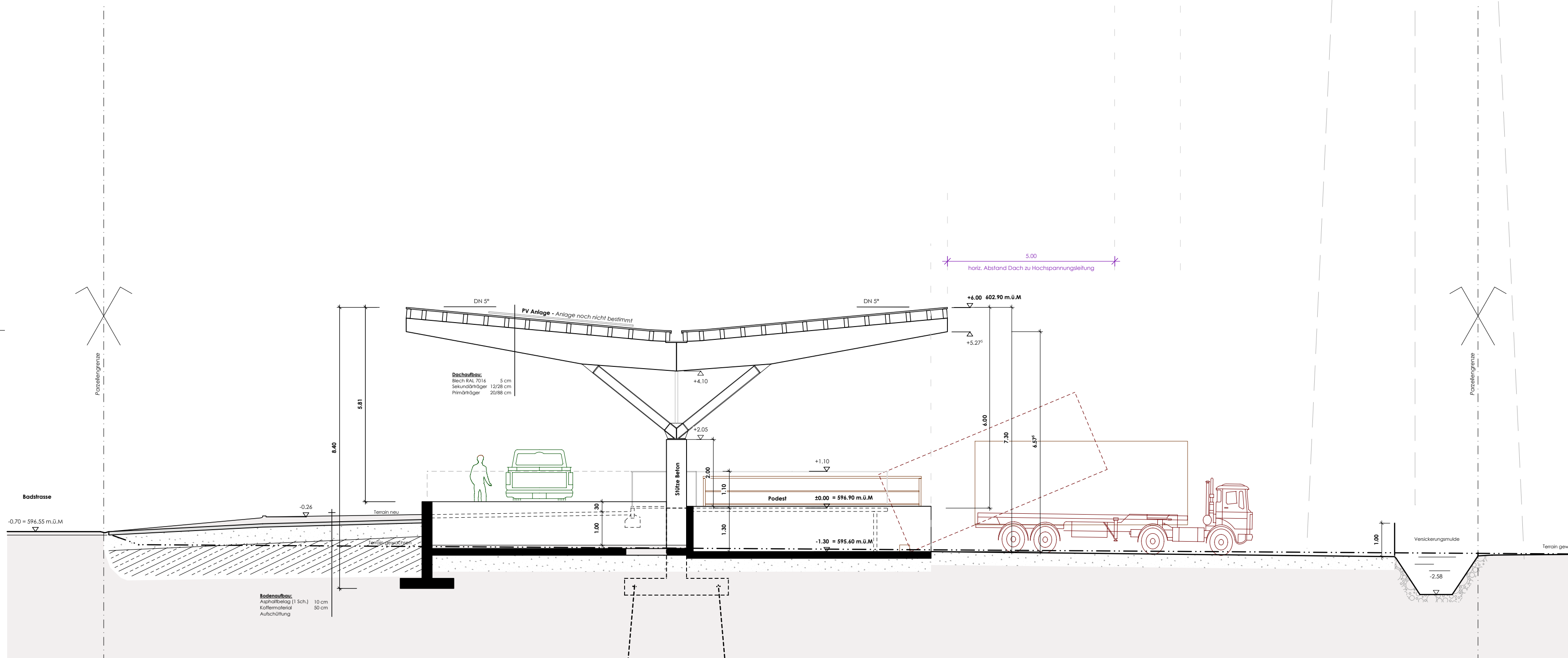
Querschnitt 2
